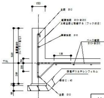
外周部断面
